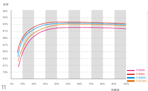
HW 1100 1-3KVA 效率曲线图
