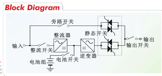
HW 1100 1-3KVA 拓扑图
